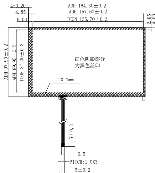
背面图
